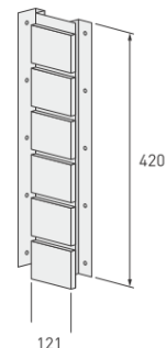
Универсален профил SB.U.
