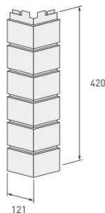
Външен ъгъл SB.NZ.
