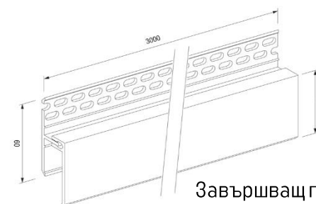
Завършващ профил FS-252... (две части)
