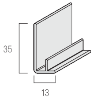
FS – 211 стартов профил
