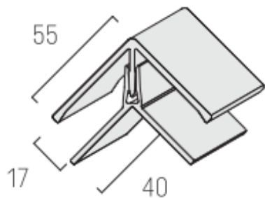
FS – 222 универсален ъгъл (2 части)
