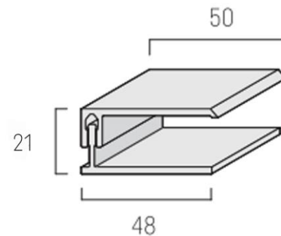
FS – 252 завършващ профил (2 части)
