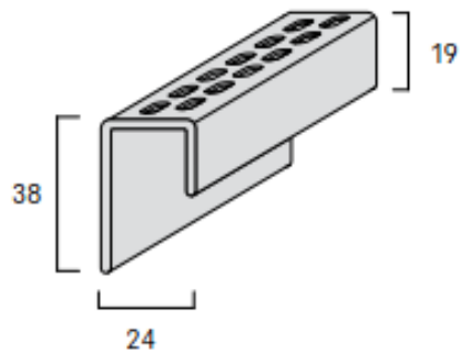
FS-261 перфориран профил
