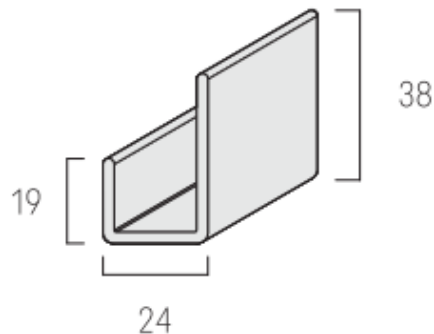
FS – 251 универсален профил
