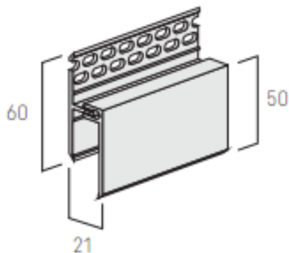
FS-262 вентилационен завършващ профил (2-part)
