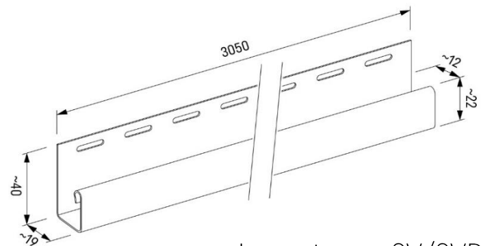
J-профил – SV/SVP-15
