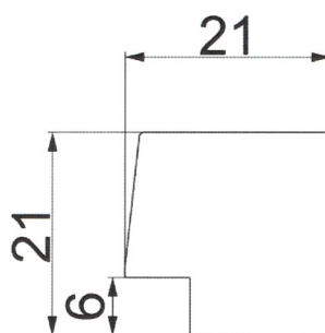
Rys. 19. Listwa końcowa M Plus Line
