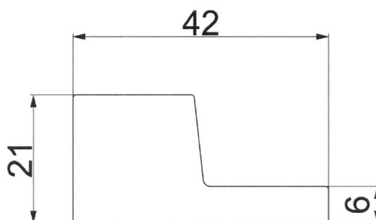
Rys. A15. Listwa startowa M Plus Line
