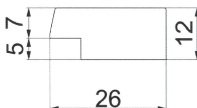
Rys. A17. Listwa końcowa R-trim M-Line
