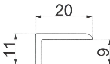
Rys. A11. Listwa uniwersalna L-XS O/W
