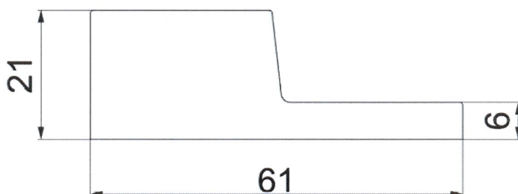
Rys. A14. Listwa startowa L-trim L-Line
